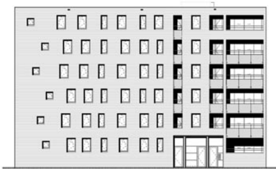
Entreegevel
