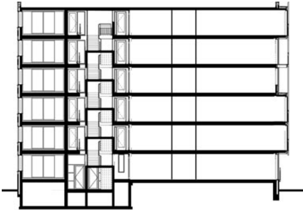
Doorsnede
