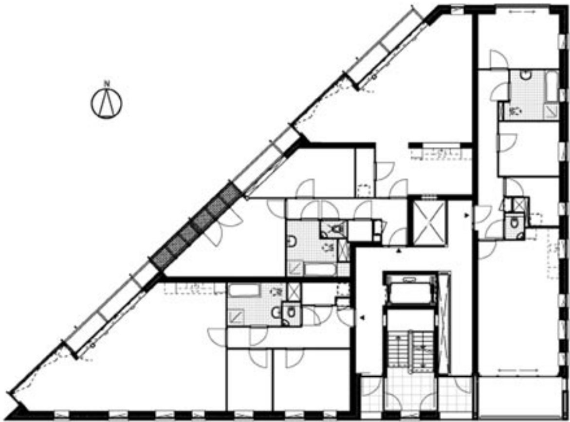
Woningplattegrond verdieping
